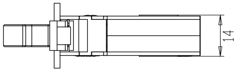
3585 双勾 衬板270长
